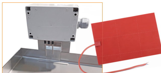
Heizkit: HEI T HER 3.0 und Heizmatten
